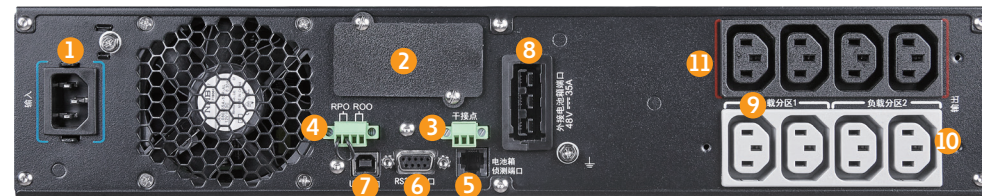
PT1K 后面板接口
