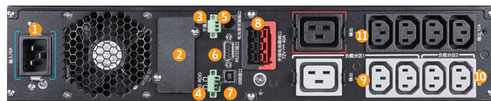
PT2.2K/PT3K 后面板接口
