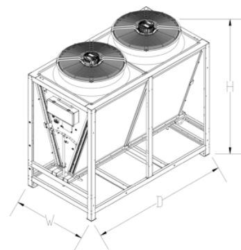
集中式冷凝器
